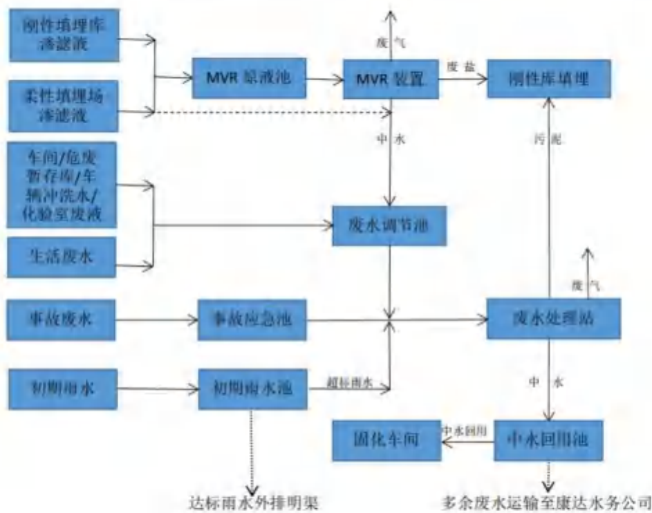
渗滤液处理工艺流程图
