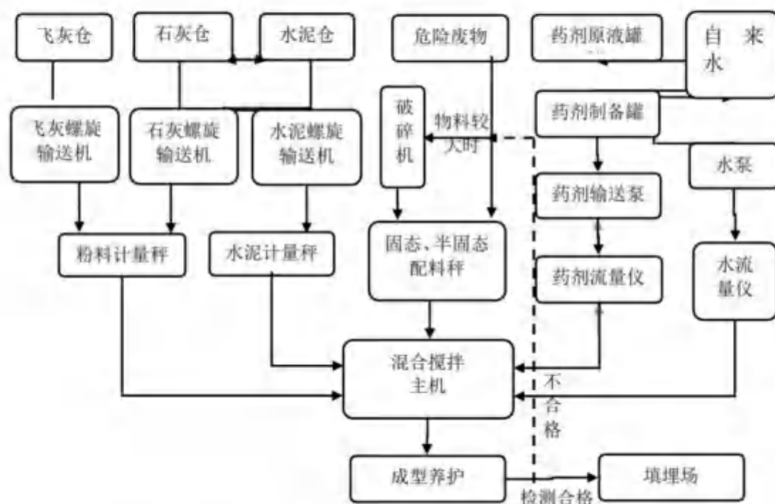
图2.3-2 固化工艺流程示意图
