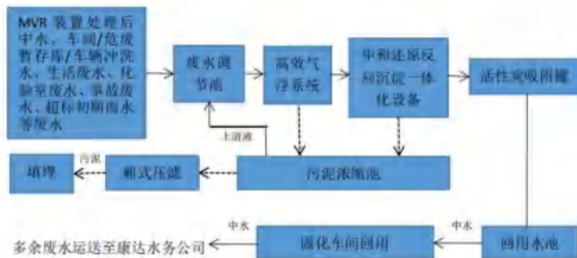
废水处理站废水处理工艺流程图
